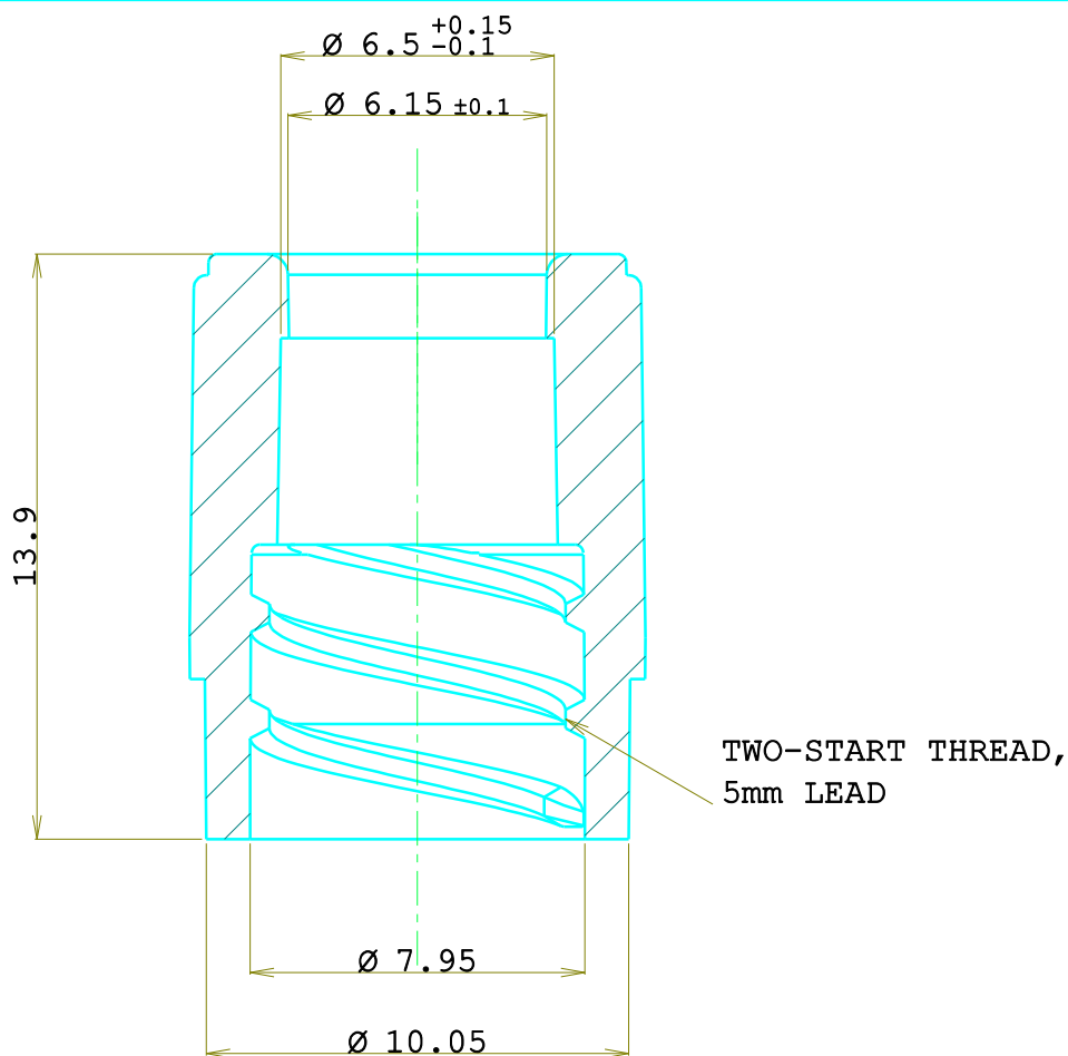
Sez. A-A
