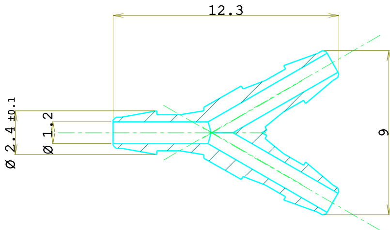
Sez. A-A
