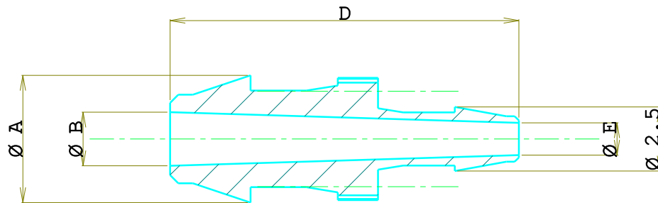
Sez. A-A
