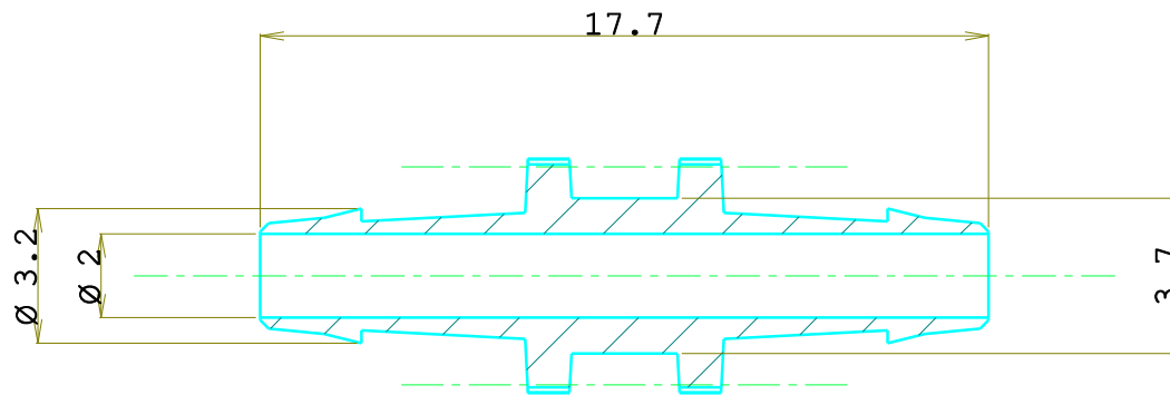
Sez. A-A
