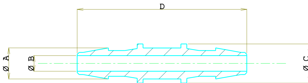
Sez. A-A
