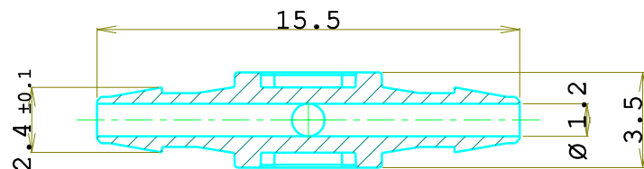
Sez. A-A
