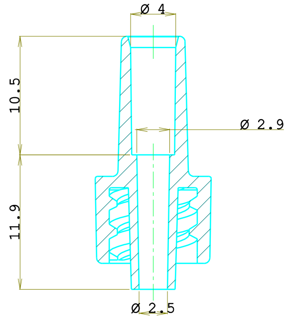
Sez. A-A
